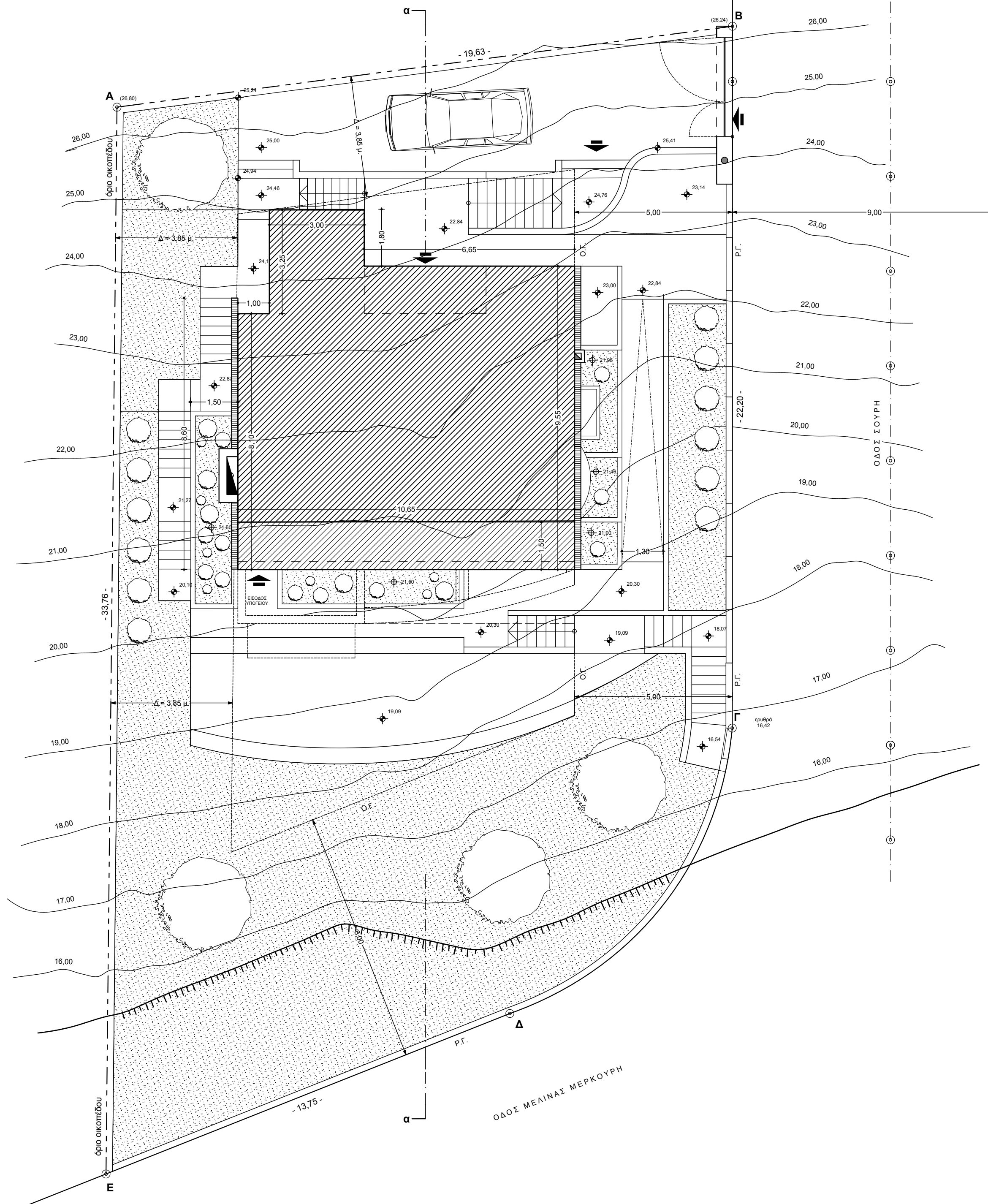
ΔΙΑΓΡΑΜΜΑ ΚΑΛΥΨΗΣ 1 : 200
