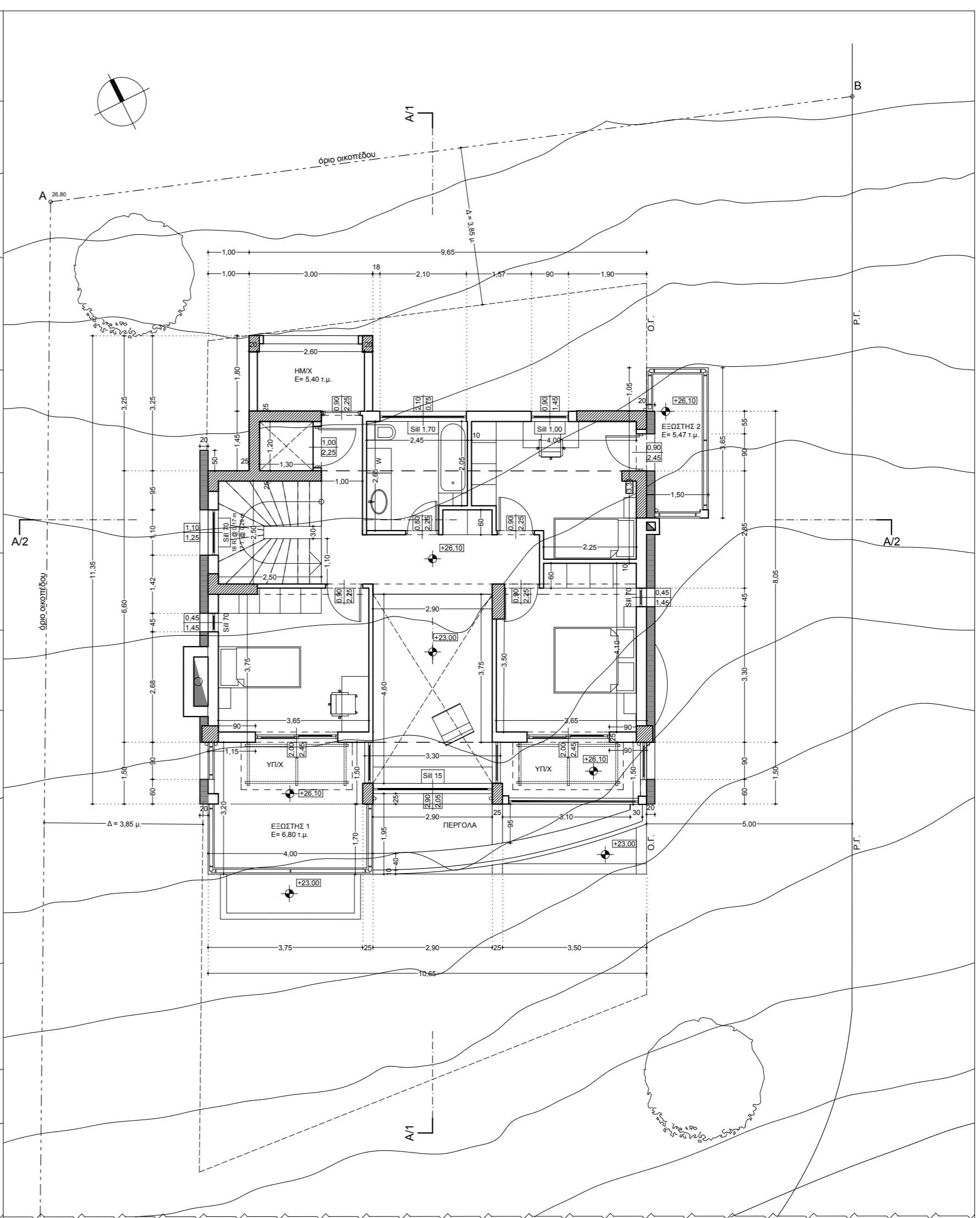
ΚΑΤΟΨΗ 2ου ΟΡΟΦΟΥ
