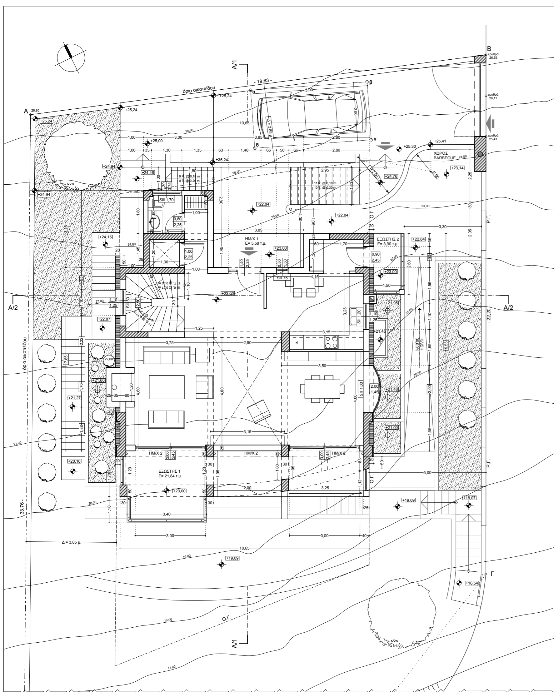
ΚΑΤΟΨΗ 1ου ΟΡΟΦΟΥ
