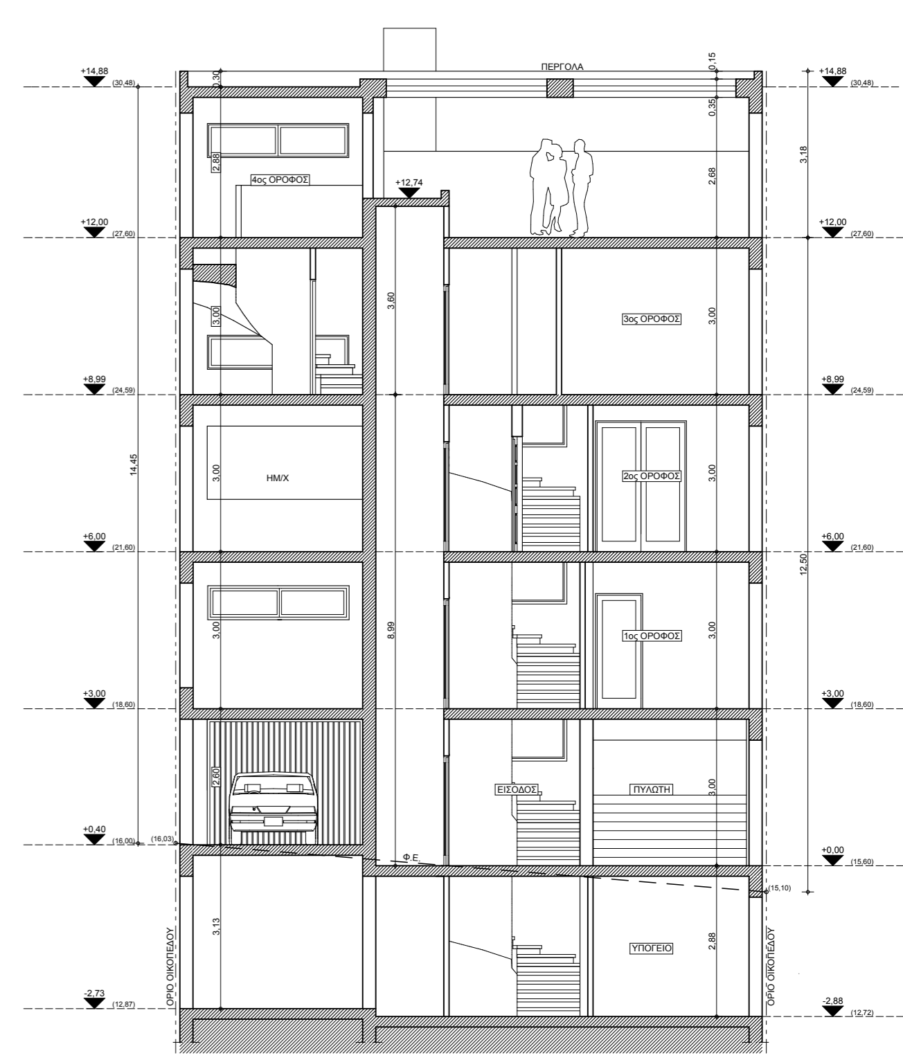
τομή A3 - A3
