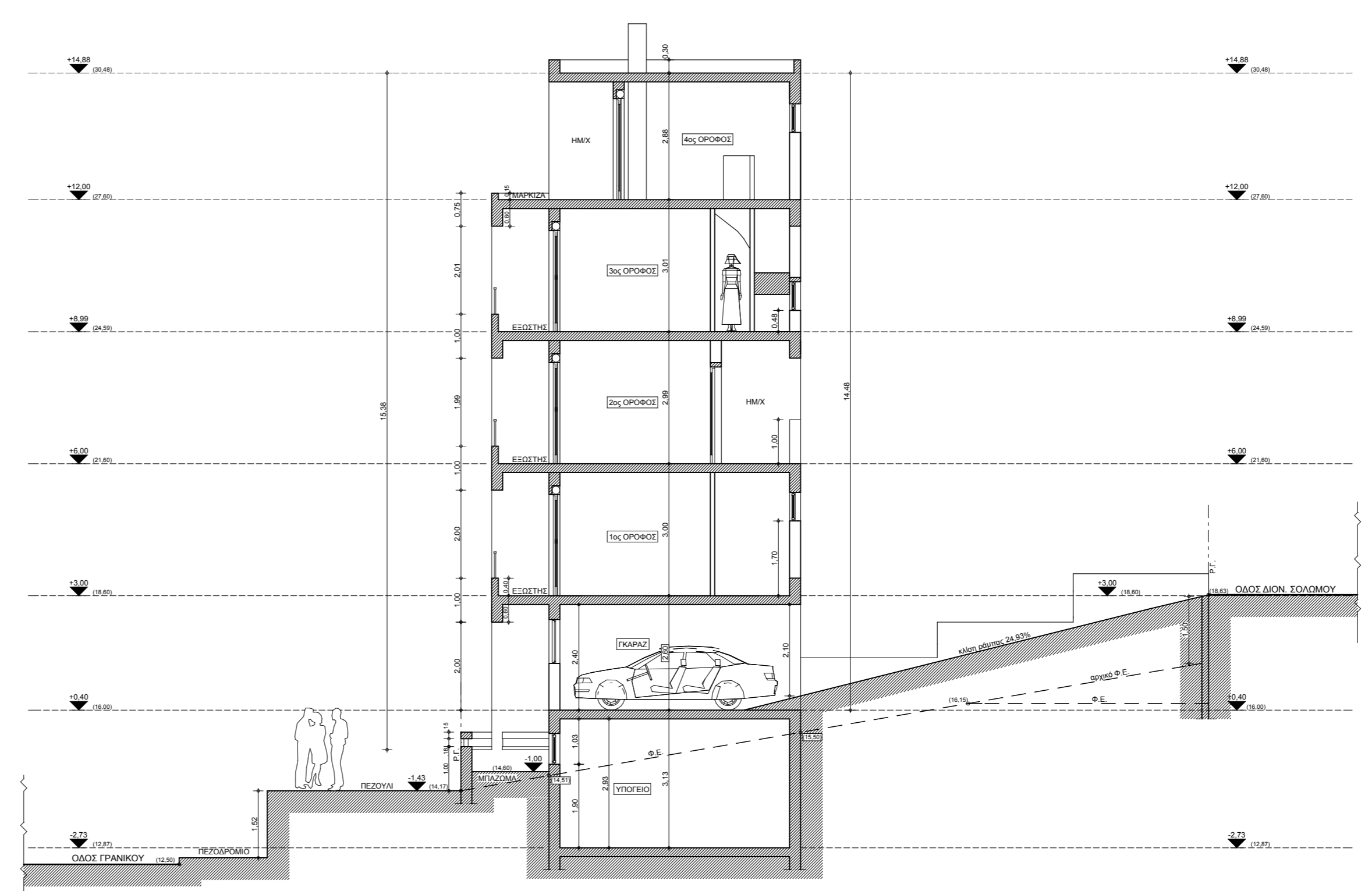
τομή A2 - A2
